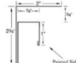
PANEL LOC PLUS F&amp;J
