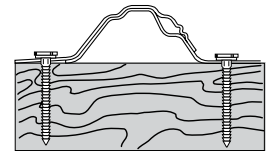
Panel-Loc Plus™ Siphon Groove
